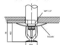
DIAGRAMA DE INSTALACIÓN
